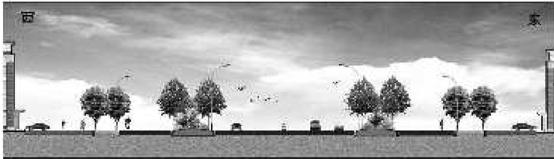
潍州路(健康街-坊子八马路)横断面图
