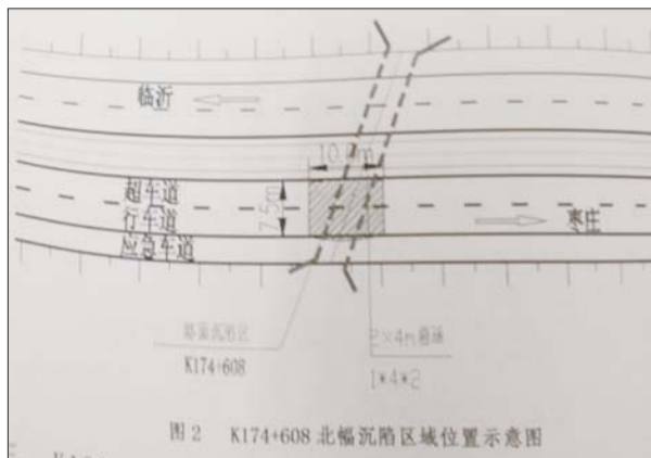
K174+608北幅沉陷区域示意图
