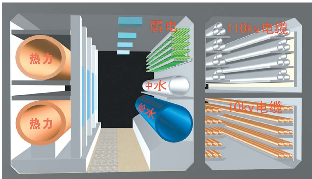
综合管廊断面(济南市市政公用事业局提供)
