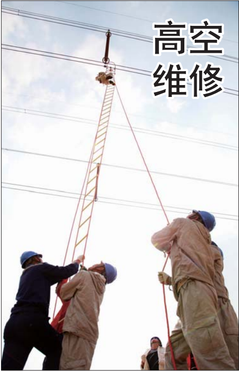
◀ 22日,威海供电公司带电作业人员在220千伏昆银线上成功实施“等电位”带电消缺作业,仅用40分钟,便消除了线路安全隐患,避免了主供线路停电给乳山市市民及企业造成的不利影响。 本报记者 许君丽 通讯员 刘中华 摄影报道
