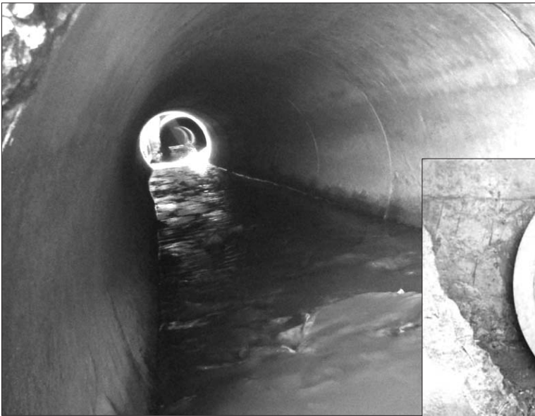
改造后的排水支管道，连接到主管道上。
