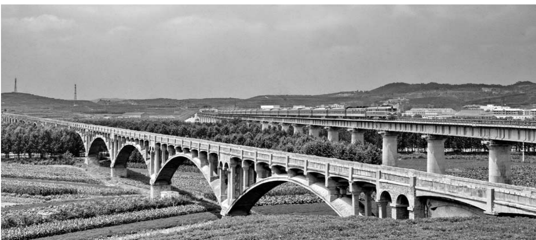
新铁路老渡槽, 这是有因有果的滋润(红旗渡槽)
