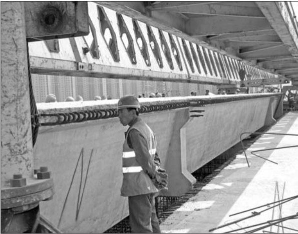
施工人员正在利用架桥机架设预制箱梁。 通讯员 付小春 黄盼阳 摄
