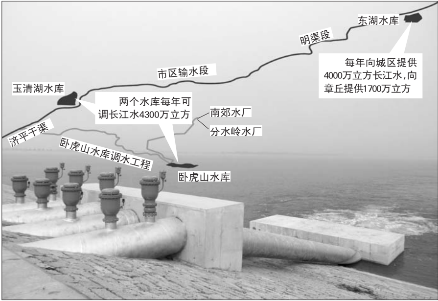
玉清湖水库引水工程近日完工,图为提水泵站正从济平干渠抽水。 本报记者 蒋龙龙 摄
