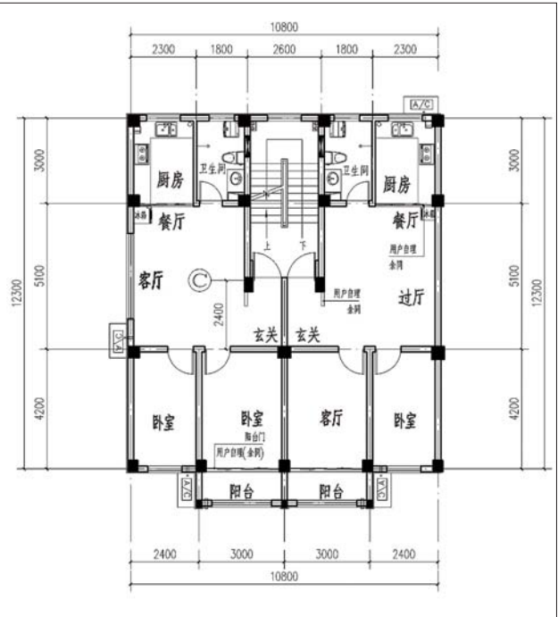
▲此次经济适用房户型模板图。
