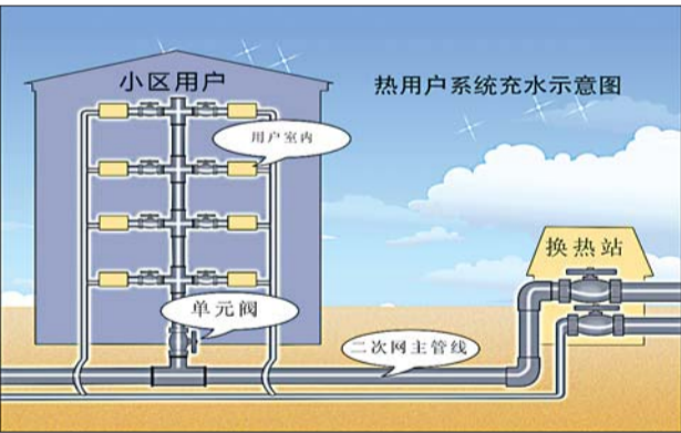
打压试水示意图
