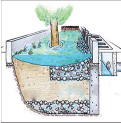
下沉式绿化带(出水)
