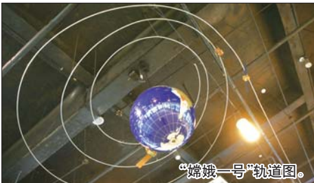
“嫦娥一号”轨道图。
