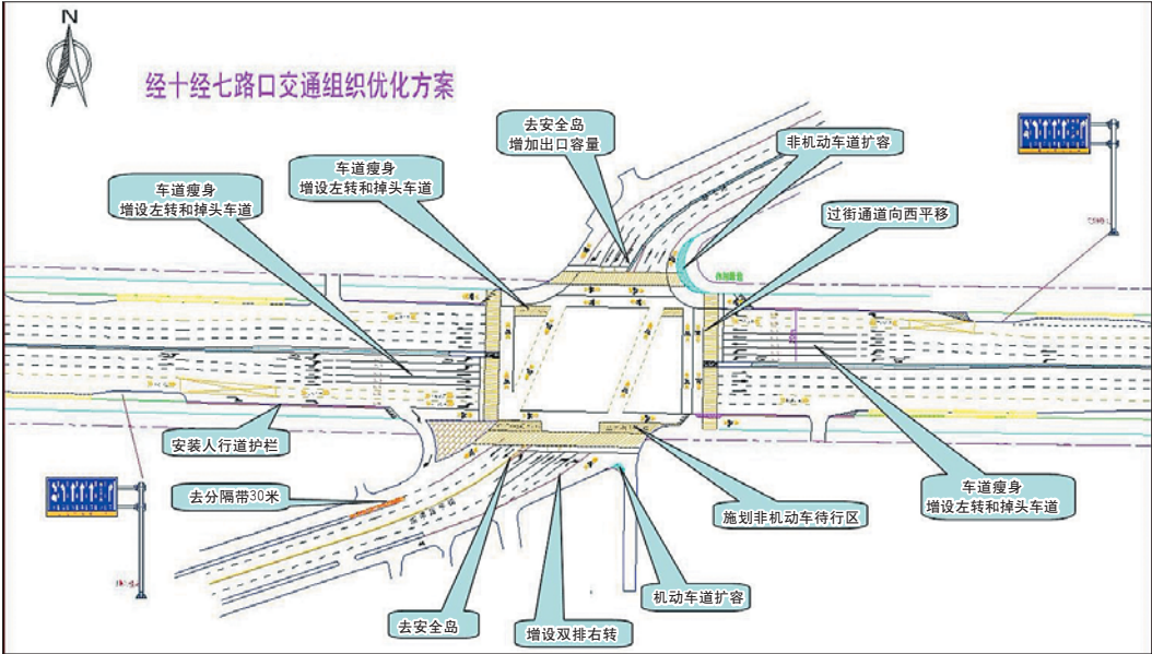
经十路经七路路口改造示意图
