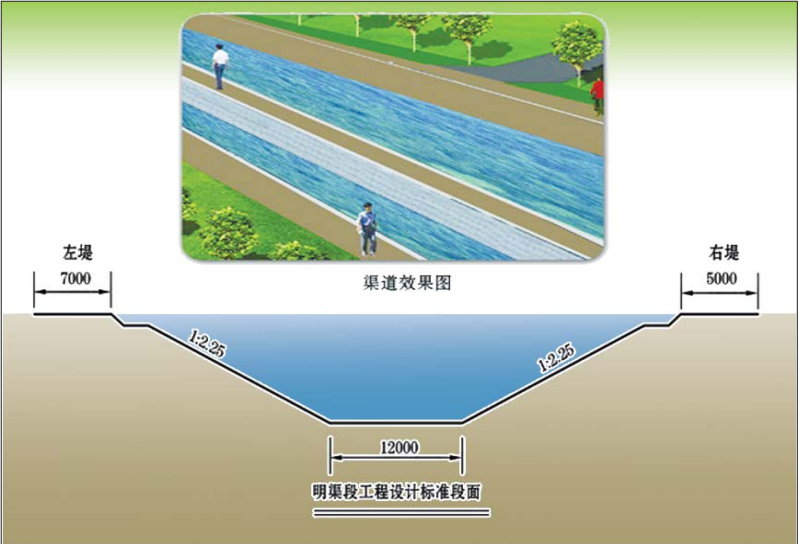
南水北调明渠段剖面效果图。
