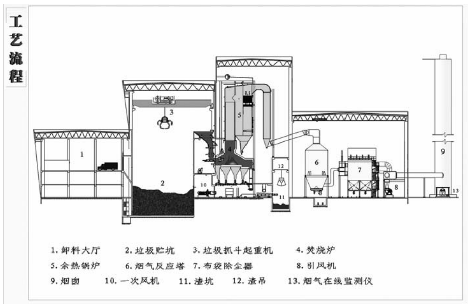
▲生活垃圾焚烧工艺流程。
