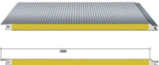
板面构造
