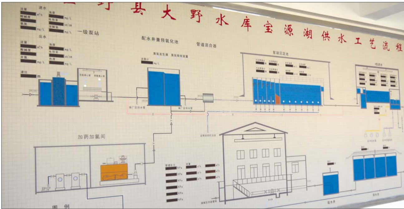
巨野县供水流程电子显示屏,可以实时显示进出水的各项参数,确保安全饮水。
