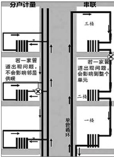
串联示意图和分户控制示意图(资料片)。
