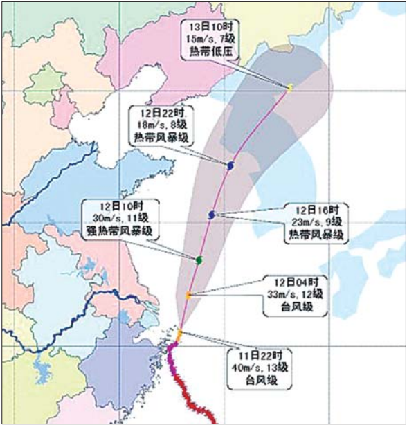
“灿鸿”未来36小时路径概率预报图 中国气象局11日22时发布
