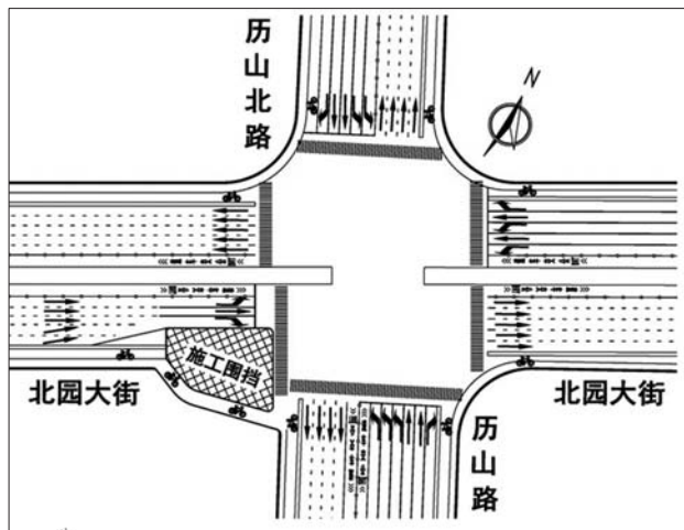
历山北路站施工交通组织方案图
