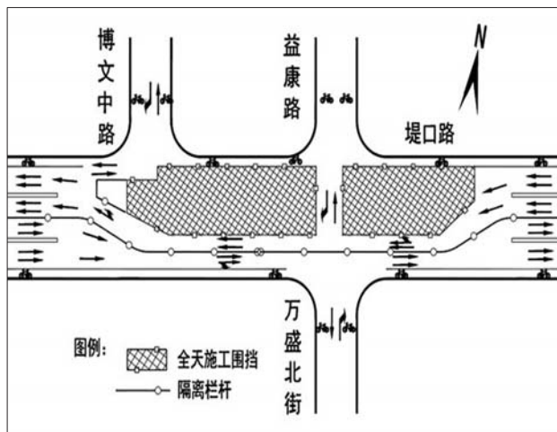
万盛北街站施工交通组织方案图
