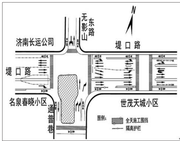
宝华街站施工交通组织方案图
