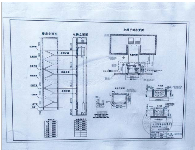
电梯加装设计平面图。
