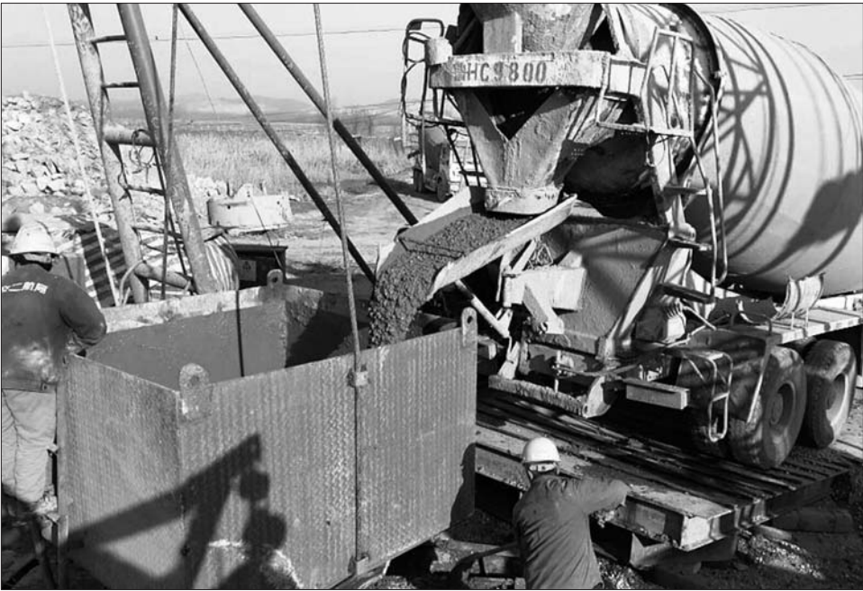
南四湖特大桥主桥首根桩基现场浇筑。
