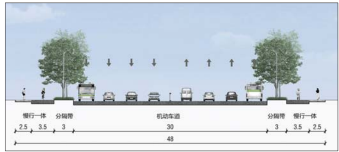
改造后道路标准横断面图。慢行一体、排水管道、照明、交通设施、道路绿化、城市家具、高压线落地改造等。昌国路以南段每侧增设10米宽绿化带。
