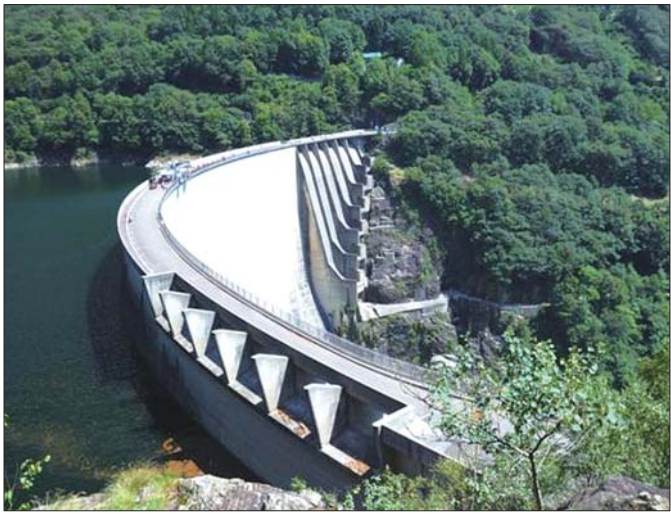
瑞士提契诺州韦尔扎斯卡大坝
