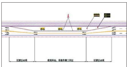
夜间施工期间交通示意图
