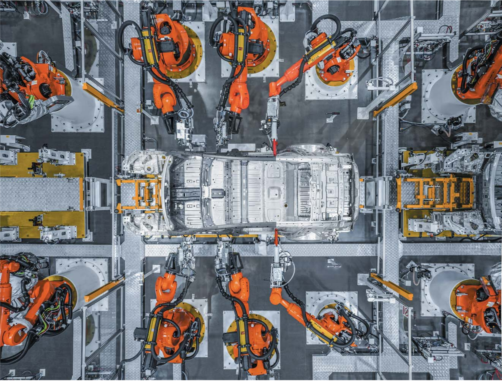
充满科技感的尊界汽车生产线。尊界超级工厂是安徽省首批筹建的零碳产业园区,也是安徽省首个5G全链路汽车制造基地。企业供图
